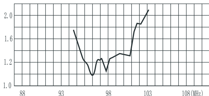
VSWR (典型值)
